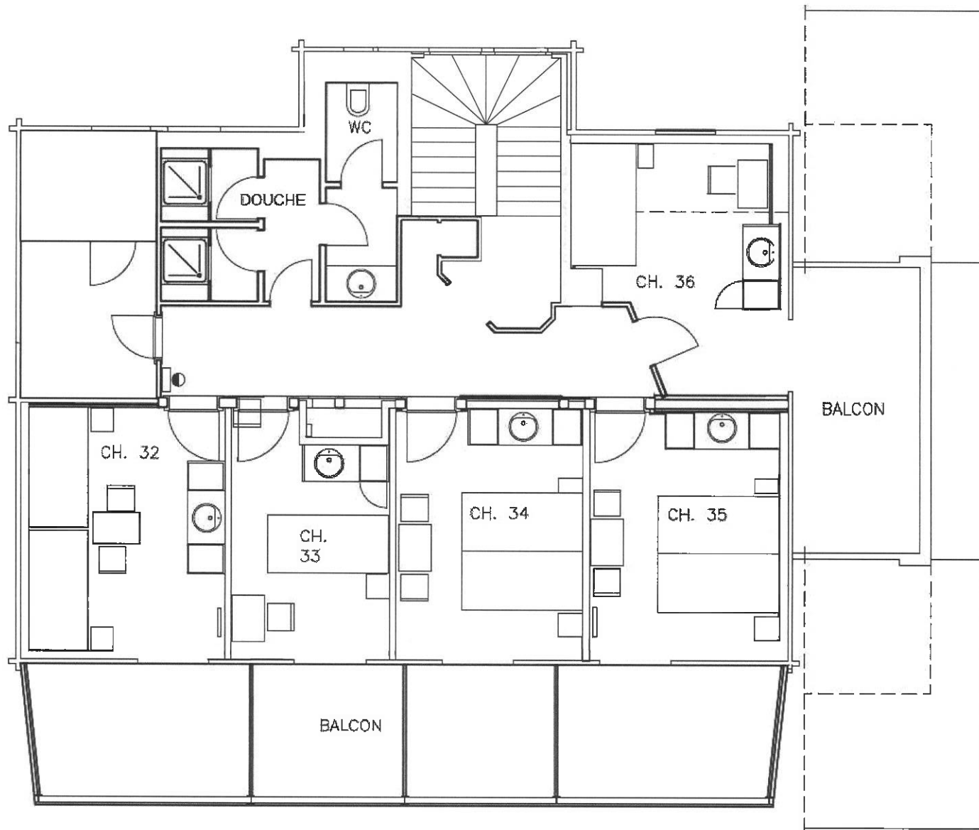
3 ème ETAGE – LES FLEURETTES
